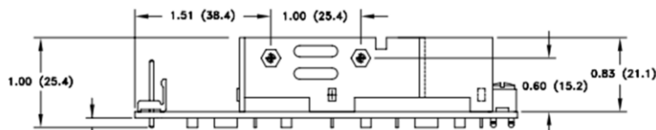
OPTIONAL CHASSIS/COVER
