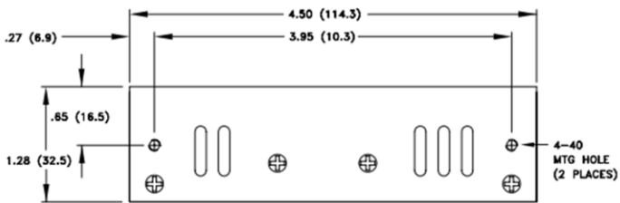
OPTIONAL CHASSIS/COVER
