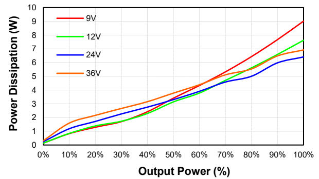
CQM60W-24D12 Pd Vs Po @25 Deg. C
