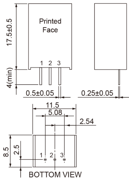
Unit : mm Tolerance : XX.X±0.5 , XX.XX±0.25
